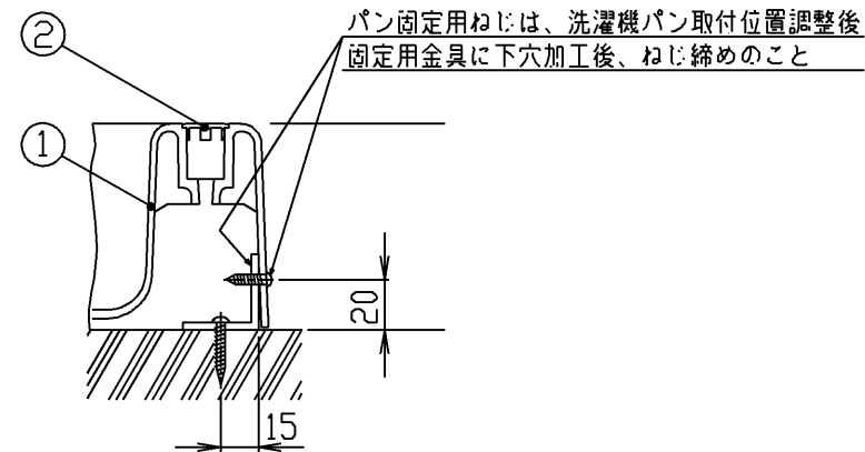
床固定部詳細(1:3)
