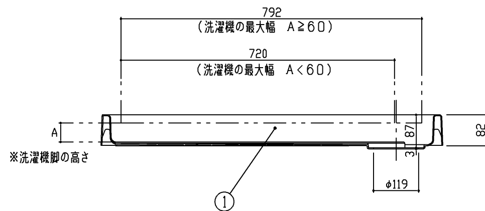
断面A-A
